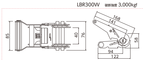
LBR300W 破断強度 3,000kgf
